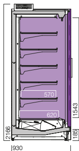
MF2 900 N CP SG 3L1 congelados frozen food
