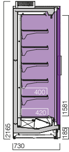
MF2 700 N CP SG 3L1 congelados frozen food
