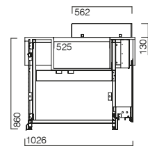
CXDSPDLS caixa padaria livre-serviço self-service bakery case casse de boulangerie libre service caja de panaderia autoservicio
