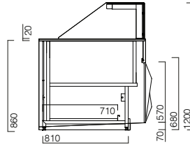
BDSNT balcão neutro com vidros counter neutral with glass comptoir neutre avec vitre contador neutral con vidrio
